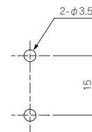
取付穴寸法図
